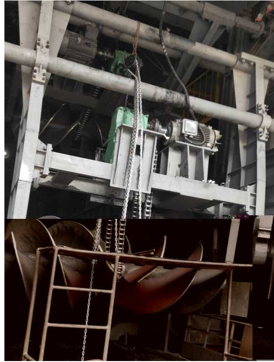
斗式卸煤机
