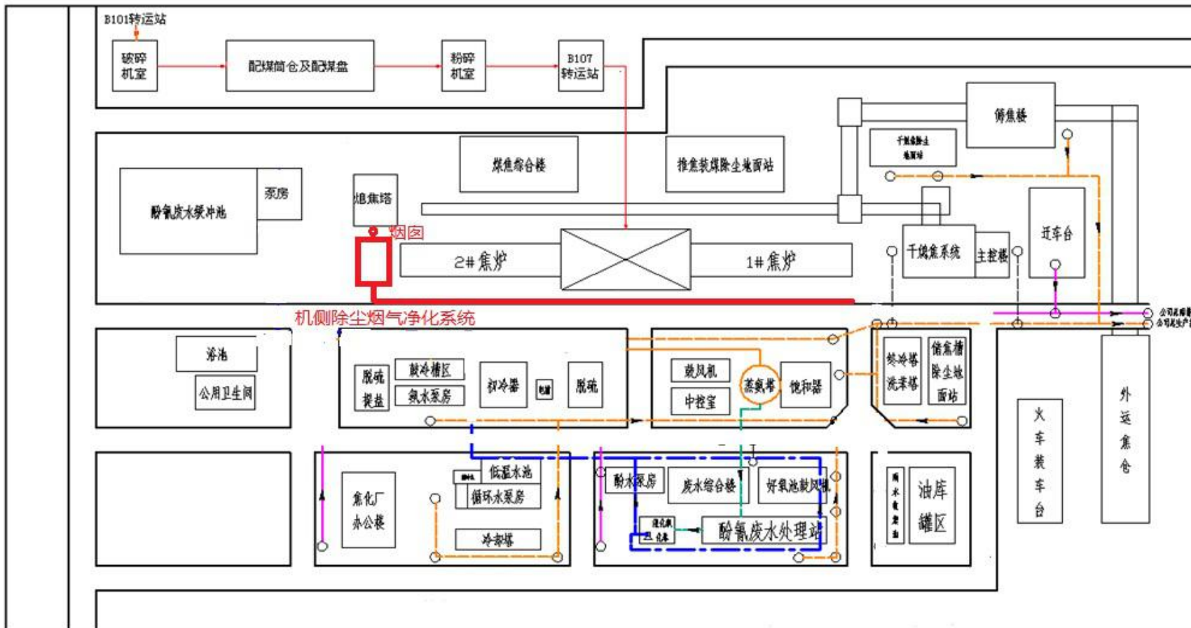
焦化厂厂区总平面图
